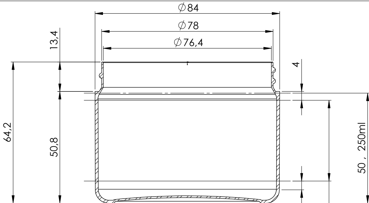
SEZIONE A-A
